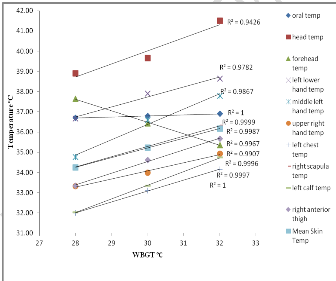
Fig. 1 Effect of WBGT on thermal parameter
