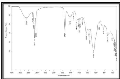
Fig 09. FTIR spectrum of F1
