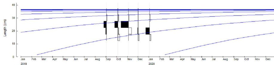
Fig. (3) von Bertalanffy growth curve.
